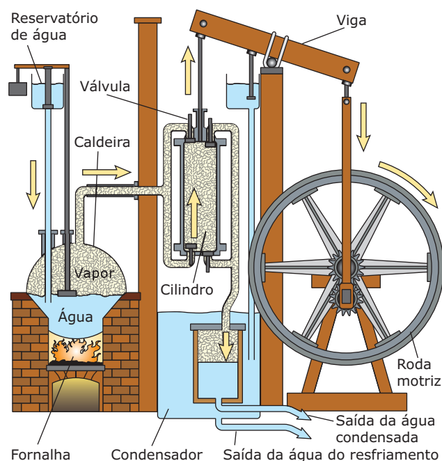
Representação do projeto de uma máquina a vapor, modelo muito utilizado durante a Primeira Revolução Industrial.
