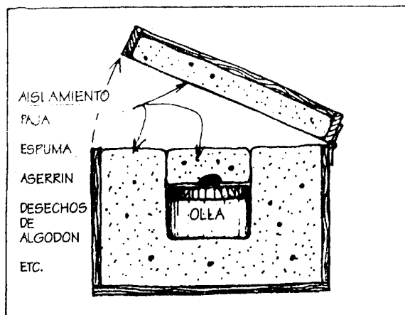
FIGURA 3.23 Olla para cocinar - aislada para cocinar alimentos lentamente (legumbres y granos)
