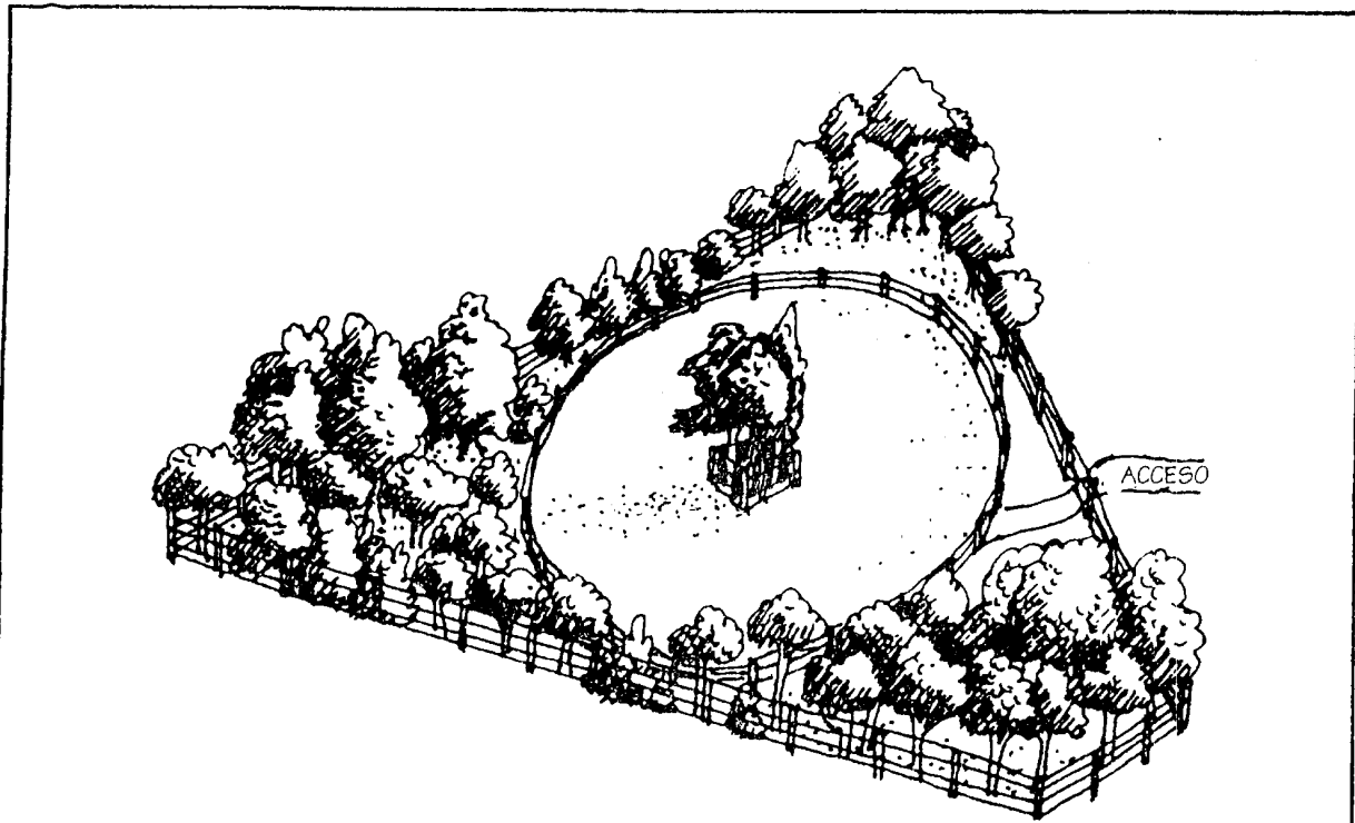
FIGURA 6.18 Permacultura rotativa: Los pastizales tienen una cerca eléctrica y se encuentran en el centro del área y las esquinas tienen cultivos de árboles. Las especies de árboles cercanas a la cerca deben ser aquellas que puedan ser rozadas o que son de sabor desagradable para el ganado.
